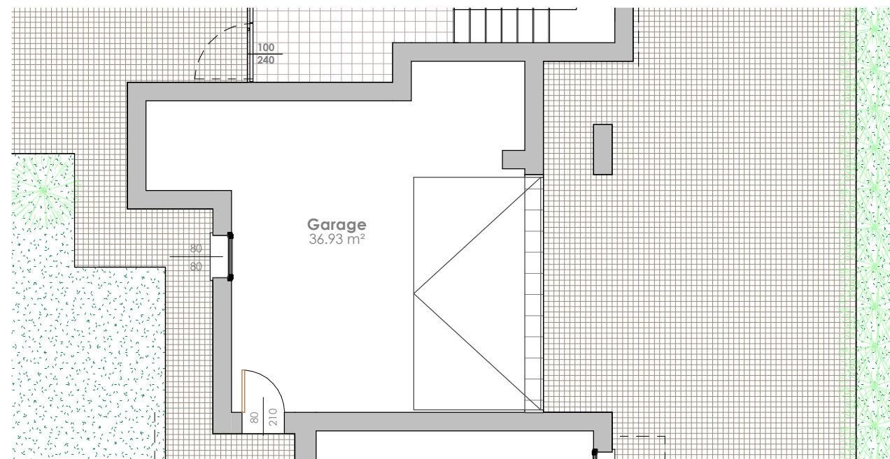
PIANTA PIANO TERRA sc 1:100
