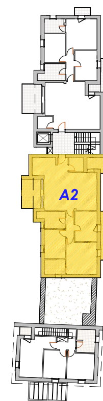
PIANTA PIANO PRIMO sc 1:500
